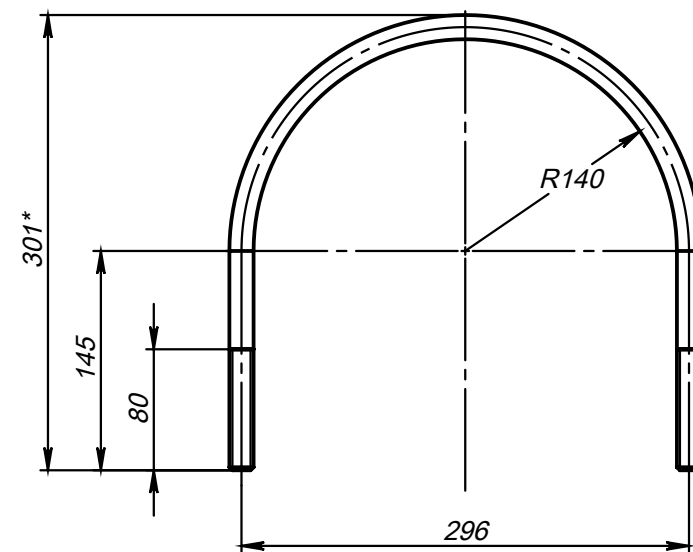
Поз.5 (Хомут)
