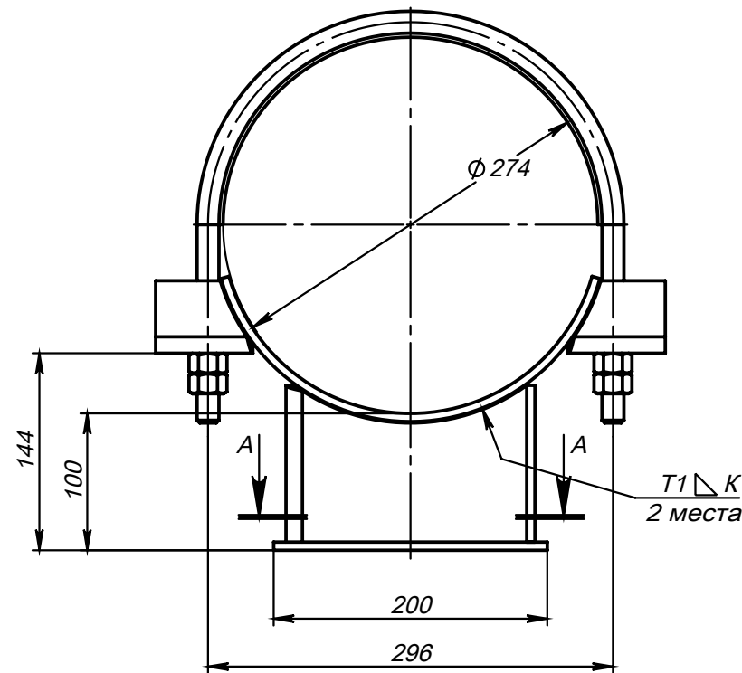
Поз.3 (Ложемент)
